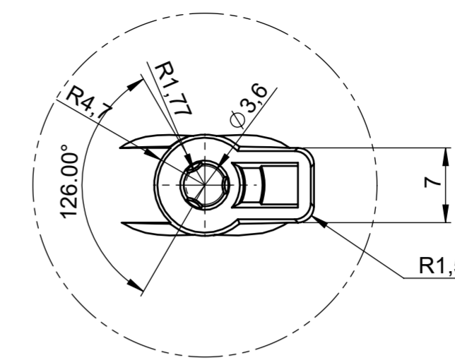
DETAIL B MAßSTAB 2 : 1
