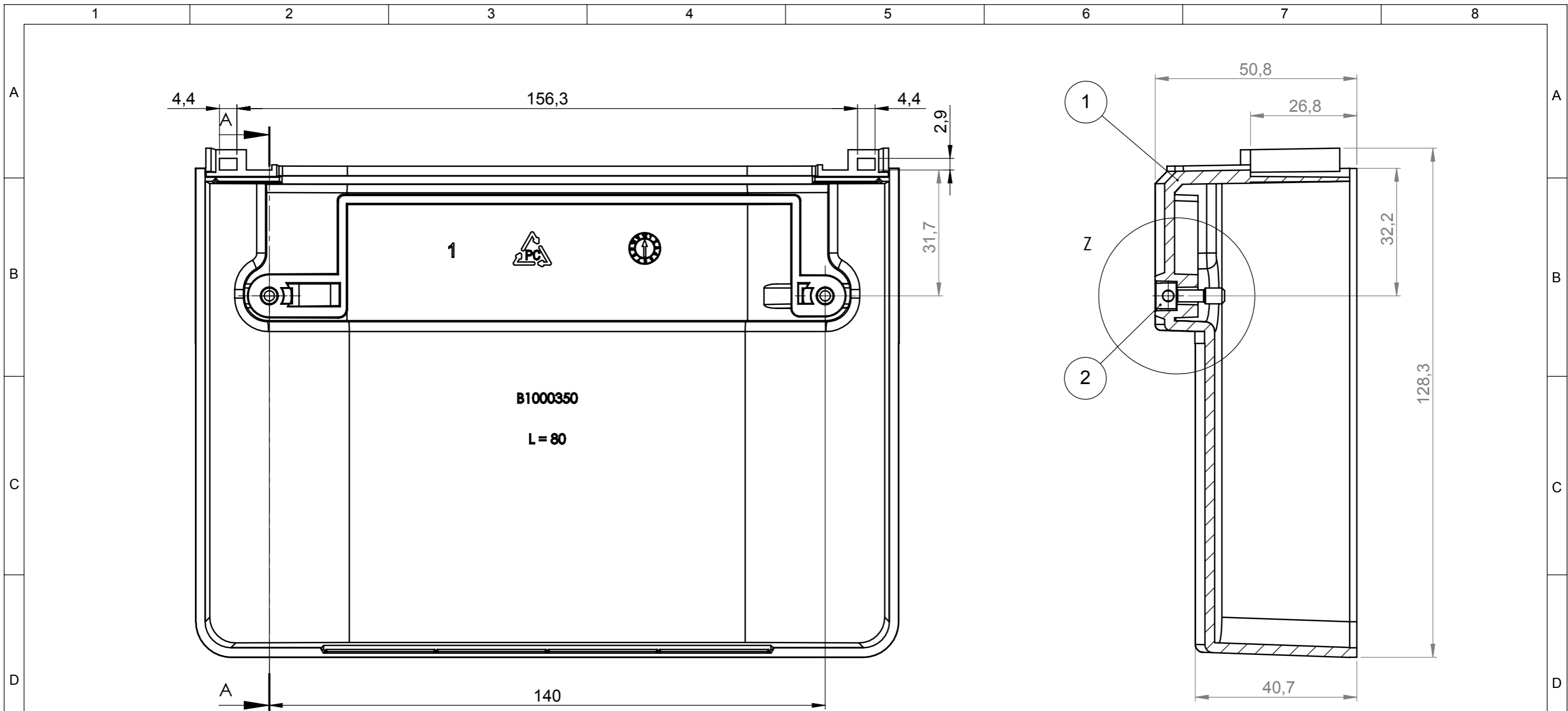
SCHNITT A-A
