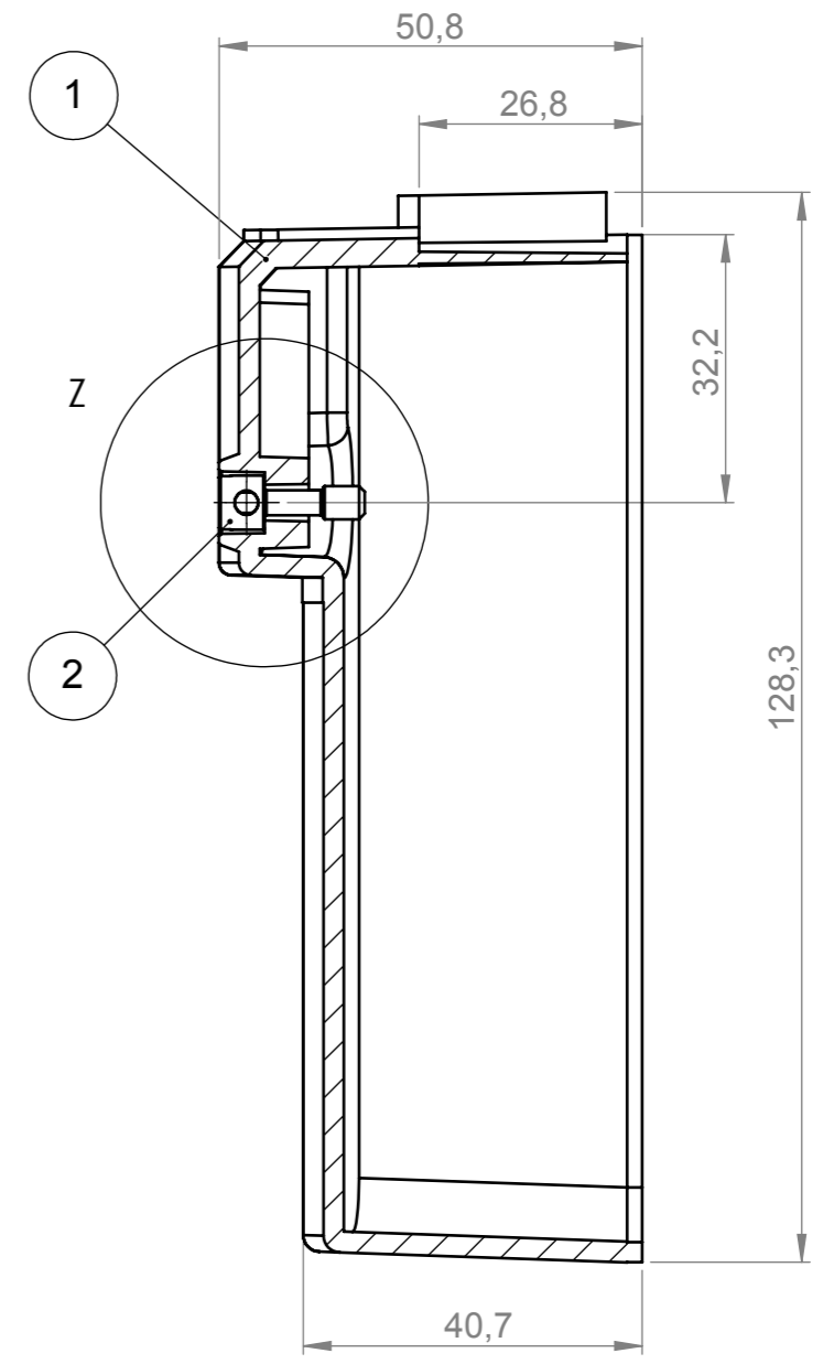
SCHNITT A-A
