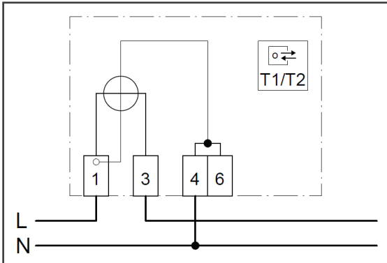
Abb. oben: Anschlusschaltbild 1100 mit Tarifschaltung, ohne Zusatzklemmen.
