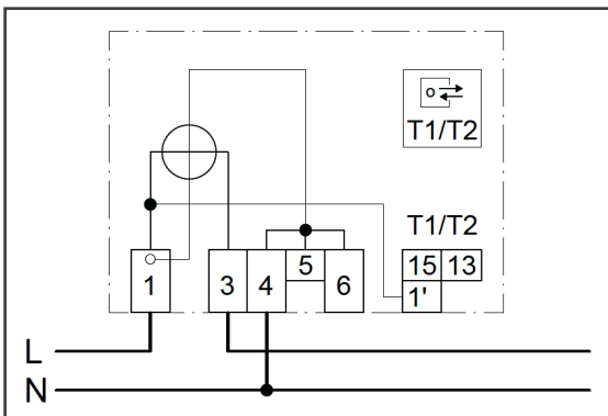
Abb. oben: Anschlusschaltbild 1102 mit Zusatzklemmen 1', 5 und mit Tarifschaltklemmen 15, 13.
