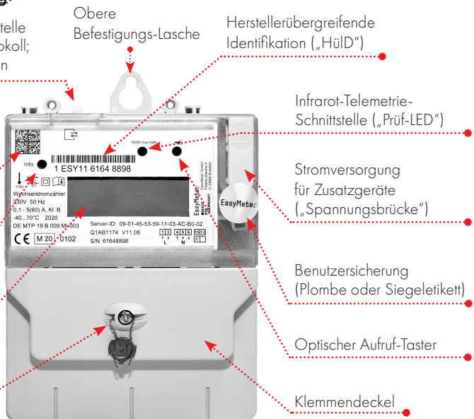
Abb. oben (Gerätebeispiel): Q1A , Typ Q1AB1174
