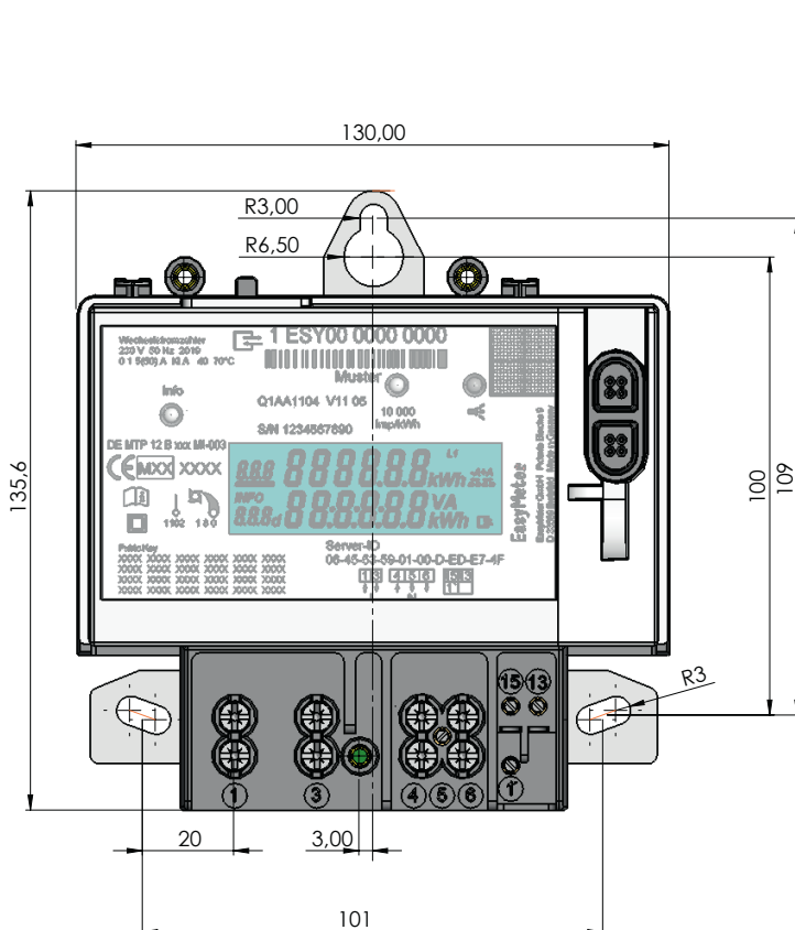
Wechselstromzähler Q1A ohne Klemmendeckel
