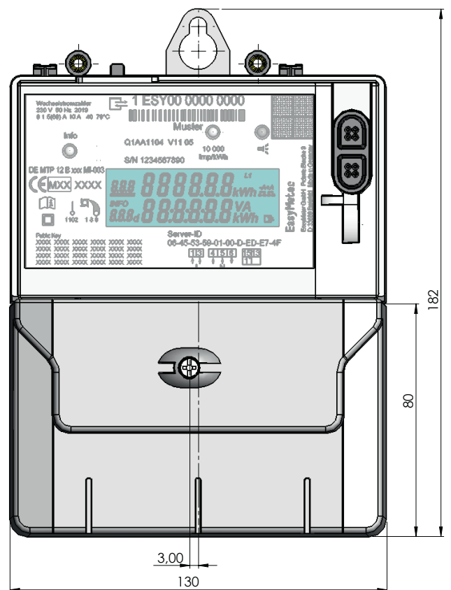
Wechselstromzähler Q1A mit Klemmendeckel
